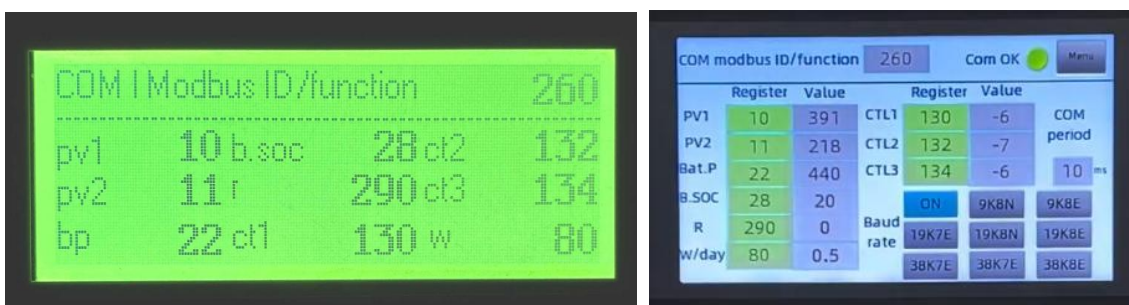
Nastavení typu modbus čtení, adresy (slave) střídače a čtení jednotlivých registrů ( na obrázku nastaveno pro Solax X3 hybrid) u staršího a novějšího typu displeje.
