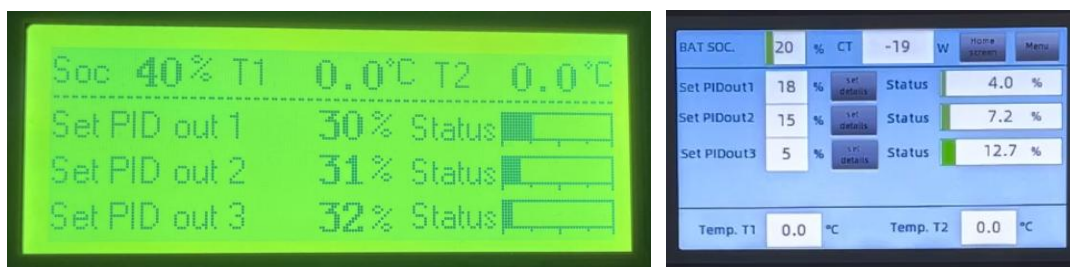
Výstupy 1-3 - obecné nastavení podle hodnoty SOC. baterie + status výstupů
