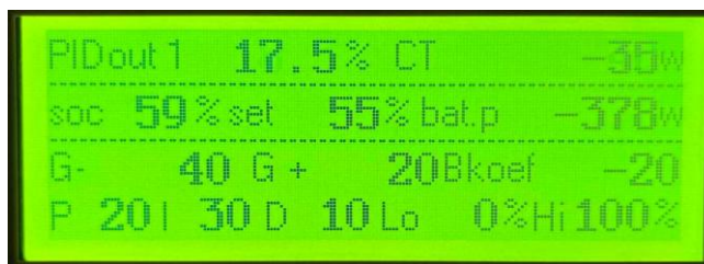
Výstup 1 - detailní nastavení PID regulace výstupu č. 1
